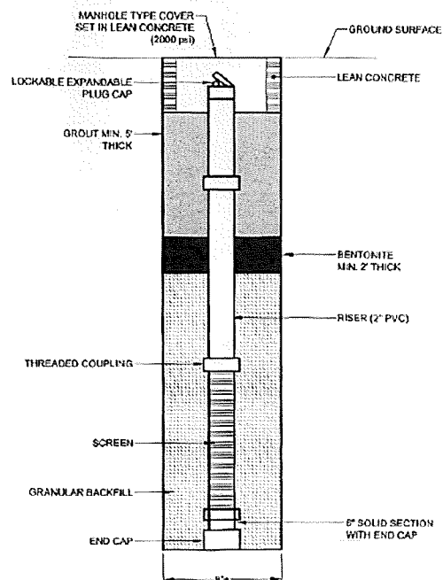
PIEZOMETER DETAIL N.T.S.
